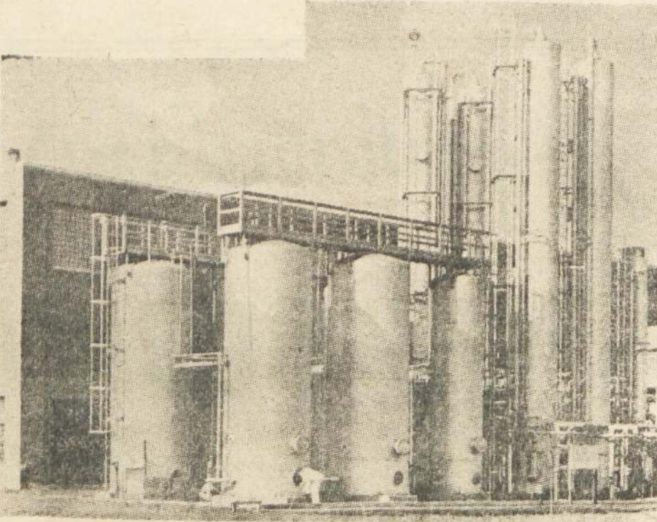
Bu keca tank ve destilatörler Terre Haute'deki penicillin fabrikasının bir kısmıdır. Bu fabrika, Birleşik Devletlerin, penicillin'i kütleli surette istihsal eden 19 fabrikasından biridir.
