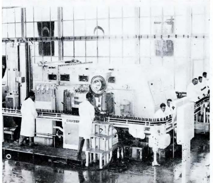
Yıkamış şişelerin doldurma ve kapsülleme makinesine otomatik olarak gidişi.
