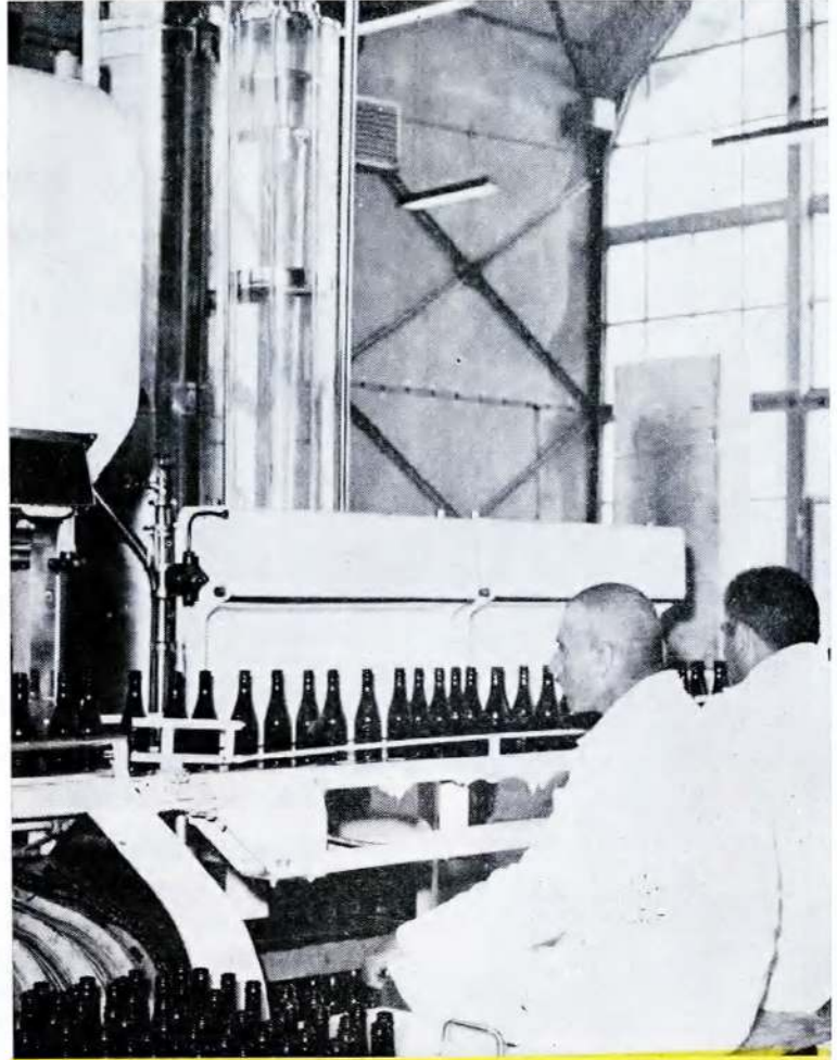
Yıkamış şişelerin bol flüoresan ışıkları altında tek tek ilk mua- yenesi. Yıkamış şişeler, bu şekil müteaddit ışık muayenesinden geçtikten ve temizliğinde herhangi bir şüphe kalmadıktan sonra madensuyu ve soda ile doldurulmaktadır.
