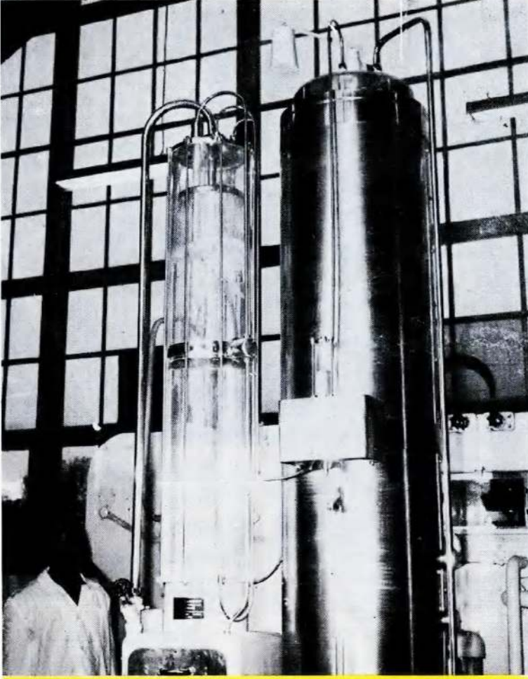
Kızılay Afyonkarahisar Madensuyu İşletmesinde kurulan yeni satüratör cihazı. Madensuyu, bu modern ve fennî cihaz içinde muayyen nispette tabii CO 2 gazıyla karıştıktan sonra şişelere inilâ edilmektedir.
