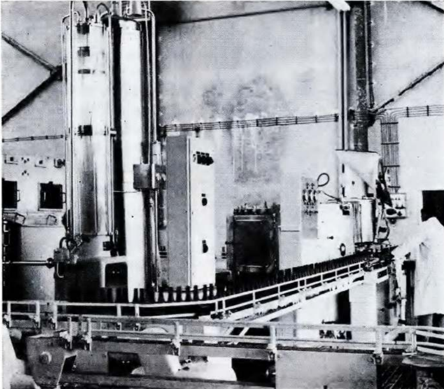
Yıkama makinesiyle doldurma ve kapsülleme makinesinin umumî görünüşü.
