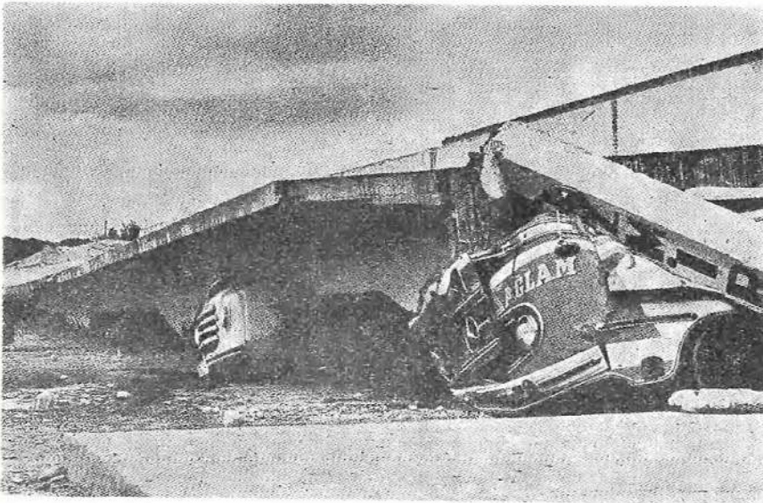
Salihlide şiddetli depremden şehir garajı da çöktü. Bu beton garajın altında kalan 18 otobüs tamamen hurdahâş oldu.
