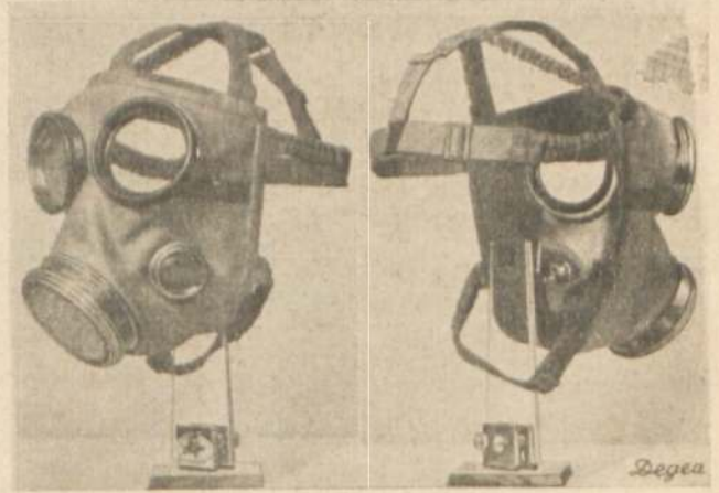
Harb maskesine benzeyen gözlük ve süpürge tertibatını havi toz maskesi
