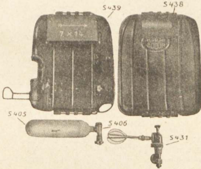
2 — Oksijen cihazının teferruatı: S 439 cihazın içi, S 438 cihazın kapağı, S 405 Oksijen bombası, S 431 otomatik dosaj manivelâ kolları.
