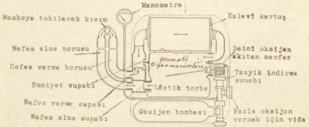
11 — Oksijen cihazı şeması.
