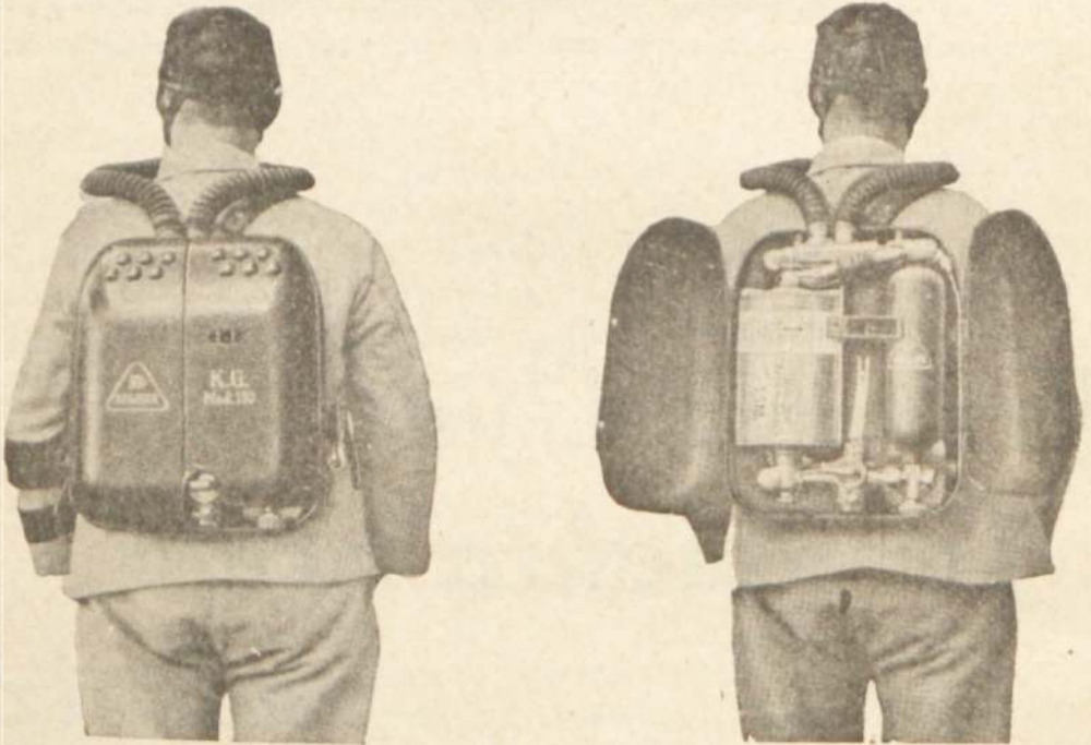
1 — Draeger fabrikasının Oksijen cihazı.
