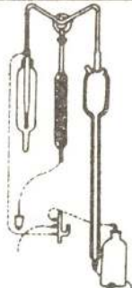
C (Karbon) tayin cihazı
